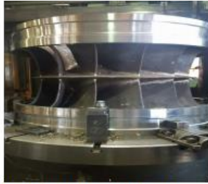
RODETE TURBINA INOXIDABLE (ACERO INOX. AISI 13/4)
